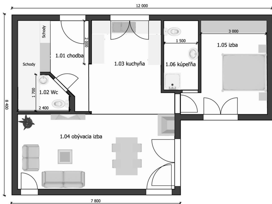
Prízemie
